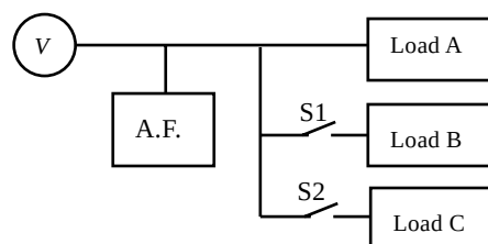
図6 負荷状態の急変時の単線図
