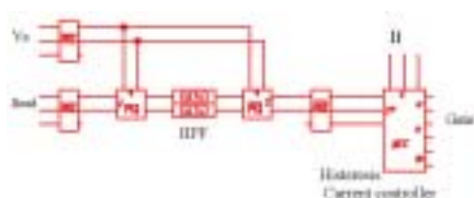
図4 AF制御ブロック
