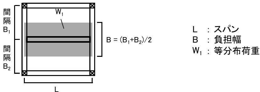
図 1 スパンと負担幅
