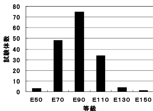
図 1 機械等級区分材の度数分布
