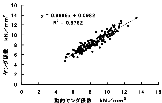
図 2 ヤング係数の相関
